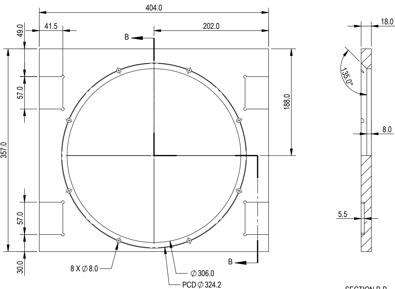
SECTION B-B SCALE 1 : 4
